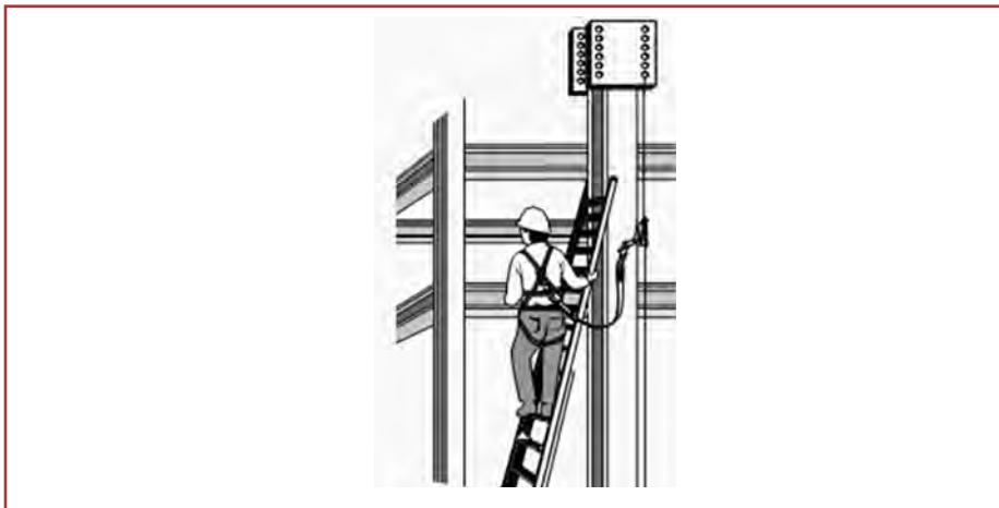
شکل ۴۳- کارگر متصل به یک طناب نجات عمودی با یک تسمه و حلقه اتصال. طناب به بالای ستون محکم شده است.
